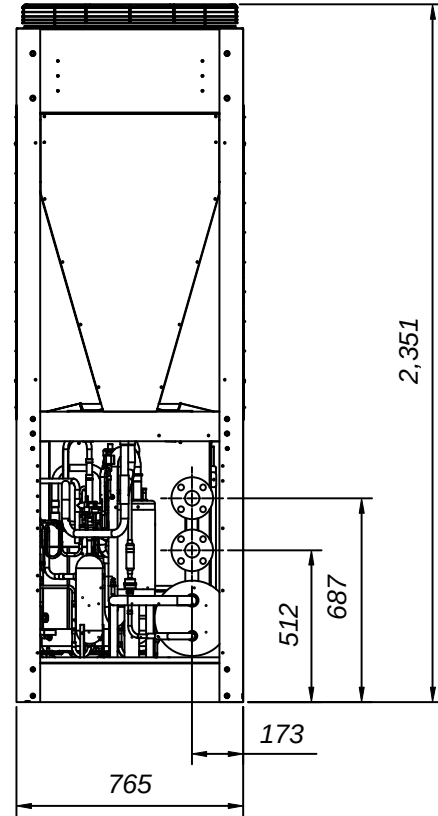
Вид сзади
